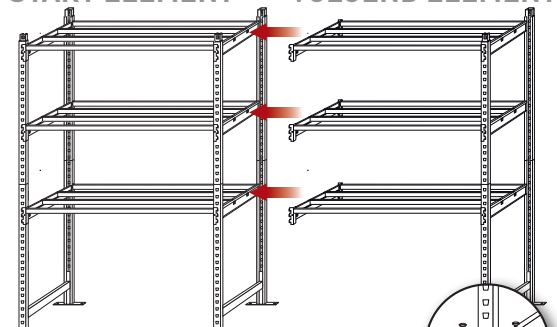
BEVESTIGINGSSYSTEEM VOOR ELKE VOET OP DE GROND
